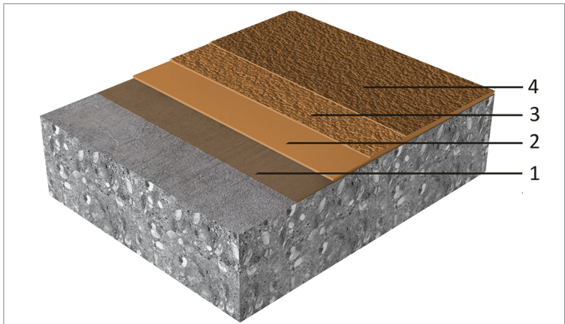
Sikafloor® Pronto RB-25 система (~3–5 мм)/Применение на поверхностях с наклоном
