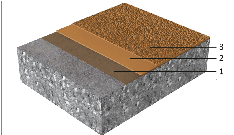
Sikafloor® Pronto RB-25 система (~3–5 мм)/Применение на горизонтальных поверхностях
